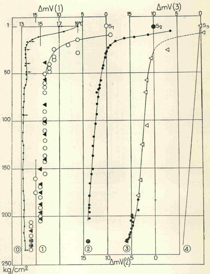
FIG. 4. — Variations relatives du pH de l'eau de mer en fonction de la profondeur par rapport aux valeurs de surface ( S_1 , S_2 , S_3 ). La pression en kg/cm^2 est en ordonnée; l'abscisse correspondant à chaque courbe donne les variations de pH en mV (voir texte).
