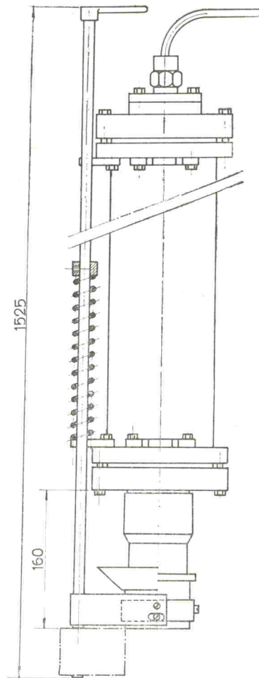
FIG. 3. — Aspect extérieur du pH-mètre (les cotes sont en mm).
